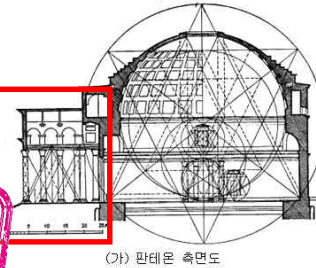
(가) 판테온 측면도
