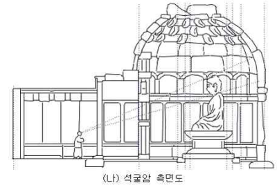
(나) 석굴암 측면도
